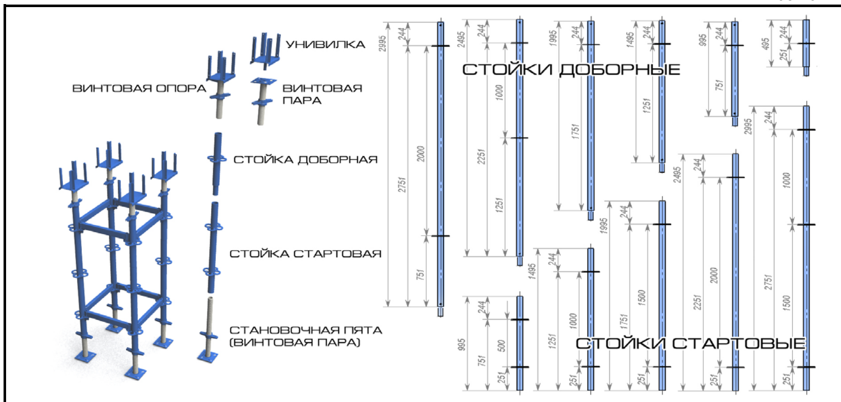
Вертикальные элементы (труба 57x2,0)
